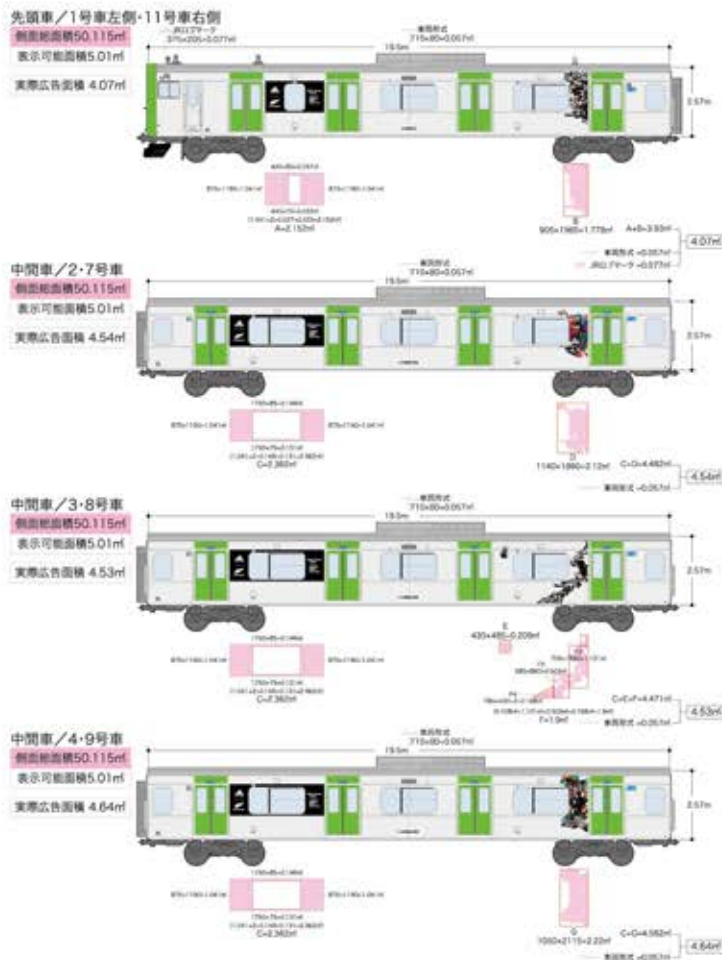
「アディダス ジャパン」山手線E235系電車 広告表示面積計算①
