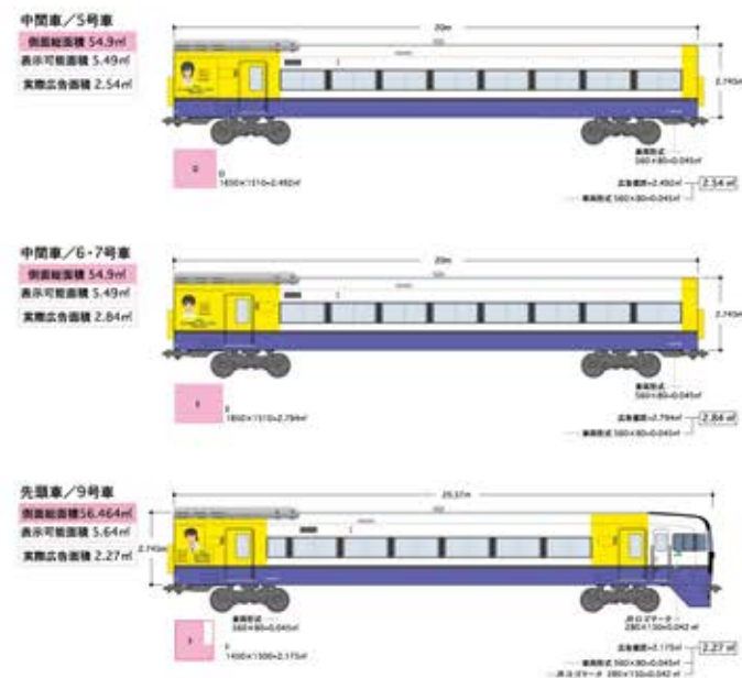
「JR東日本千葉支社営業部」255系電車 広告表示面積計算②
