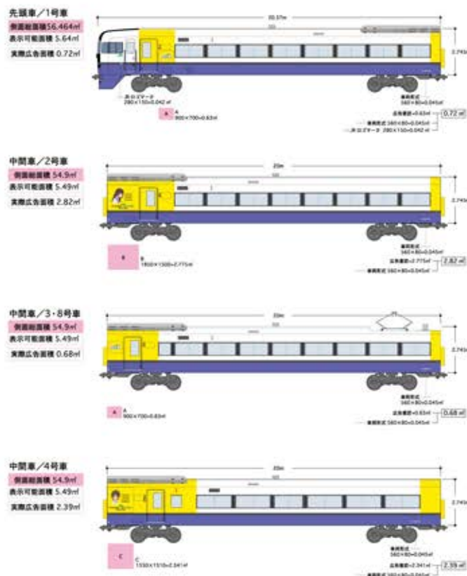
「JR東日本千葉支社営業部」255系電車 広告表示面積計算①
